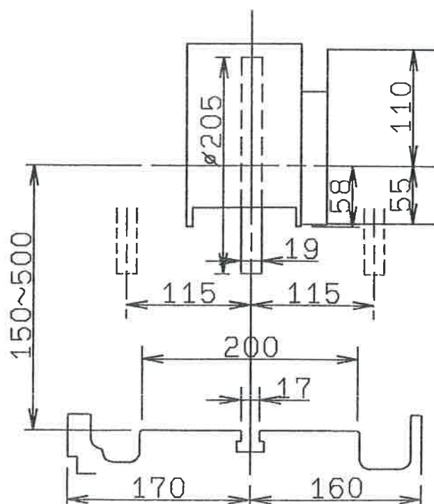
加工範囲図
